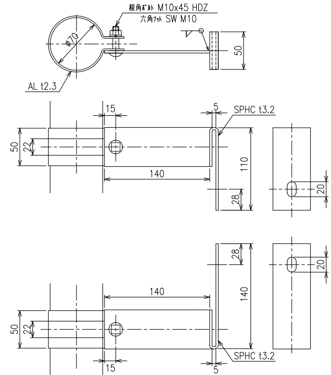
取付金具 S=1:5
