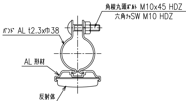
A - A' 断面図 S=1:3
