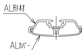
B-B' 断面図
