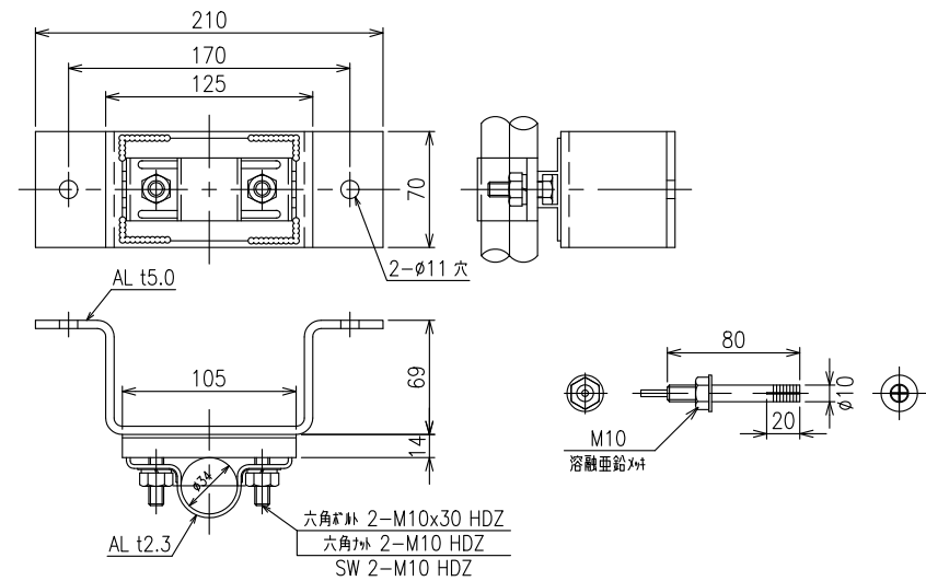
壁面金具詳細図
