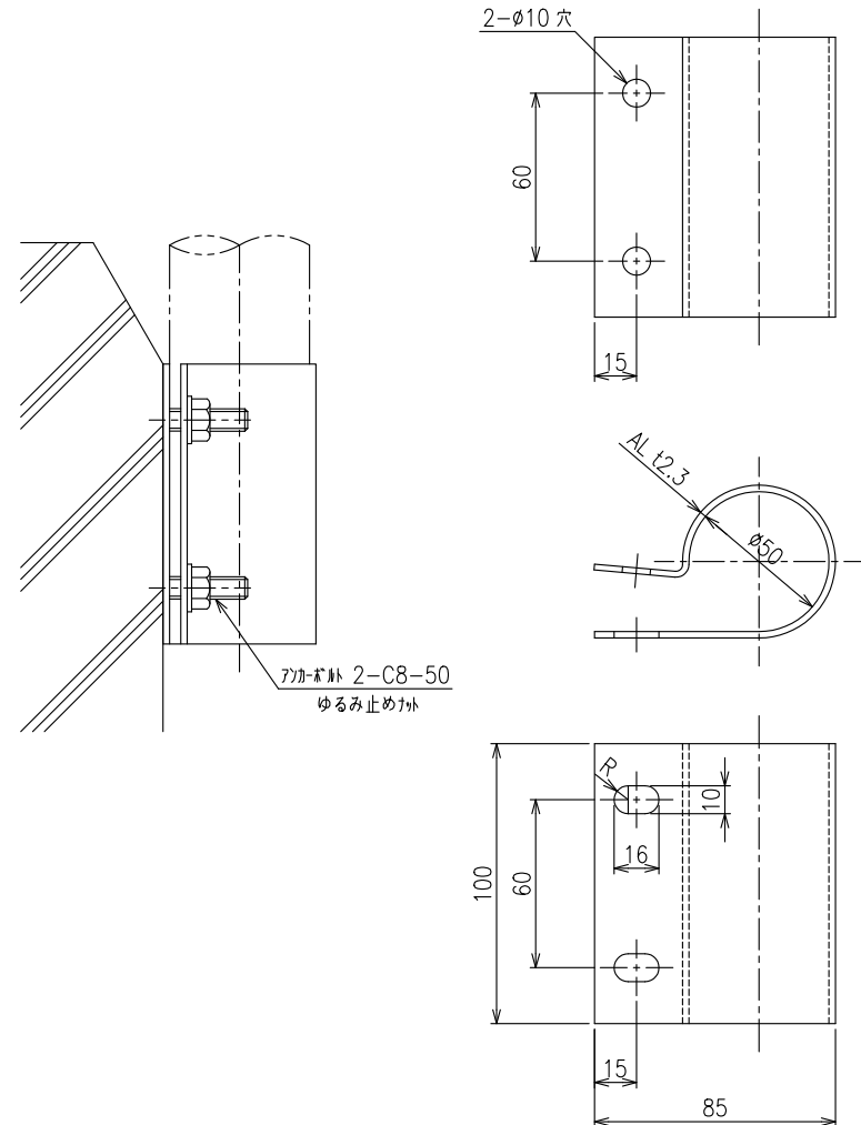
金具詳細図 S=1:4
