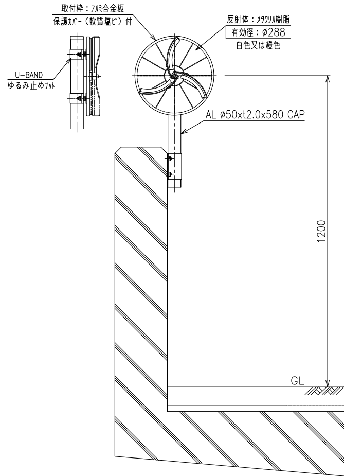
設置図 S=1:15
