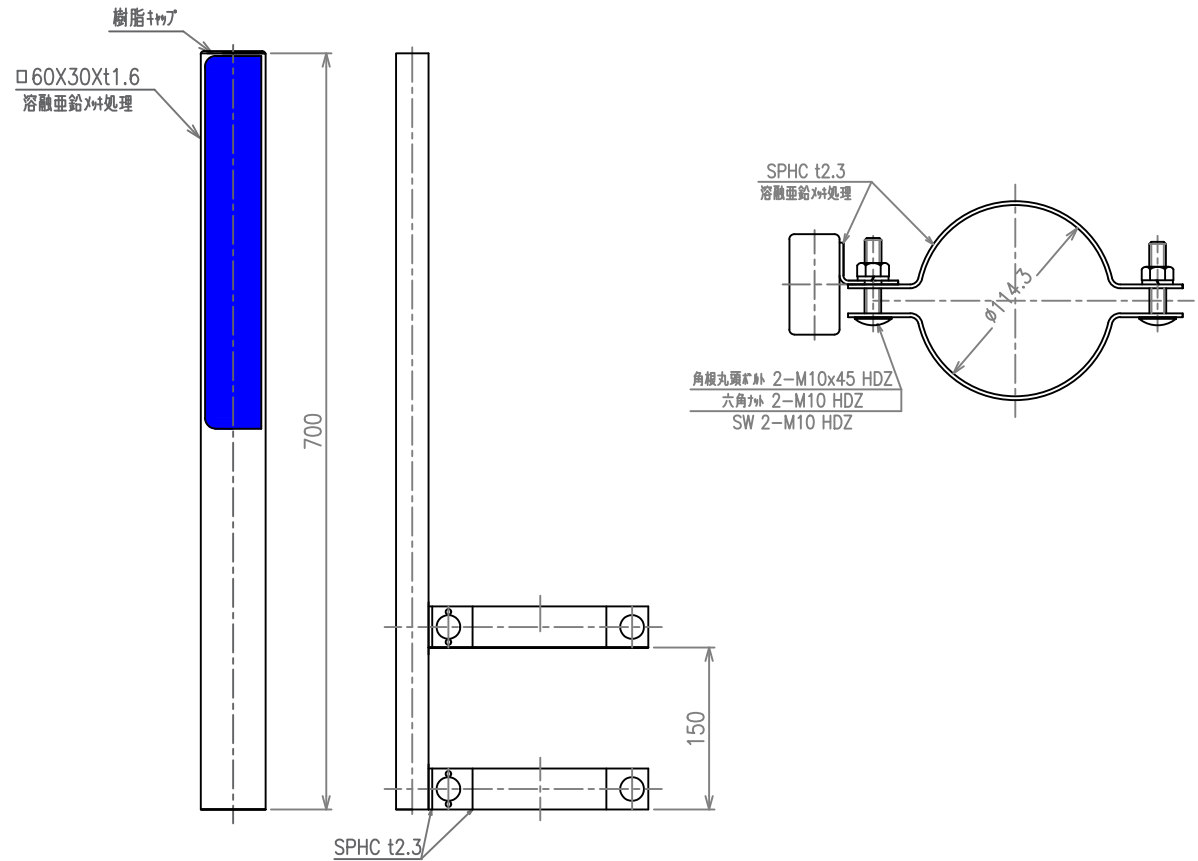
詳細図 S=1:7
