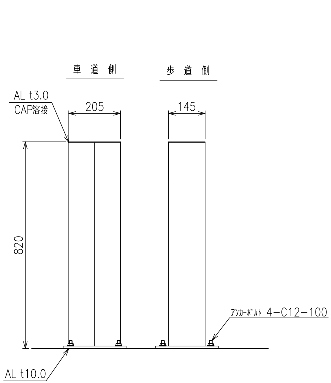
設置図 S=1:15
