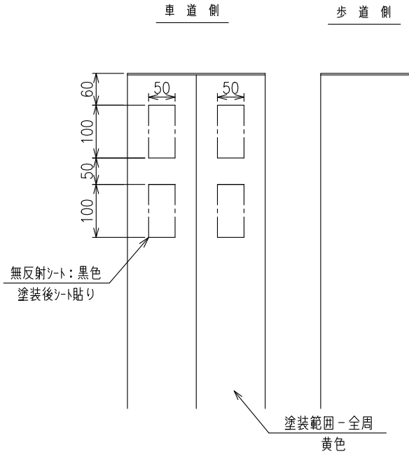
標示面詳細図 S=1:10
