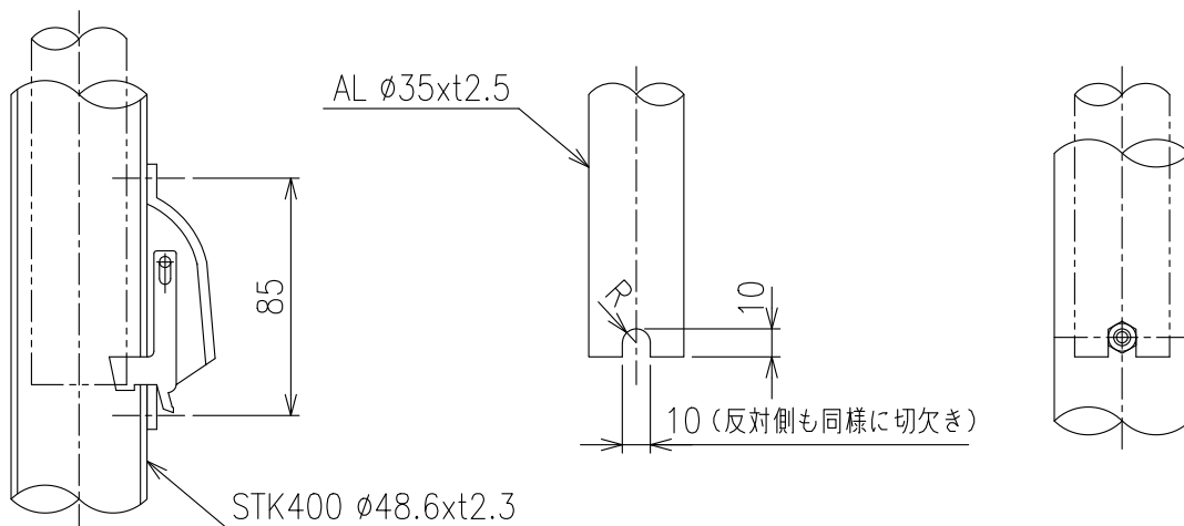
フワタッチ金具 詳細図
