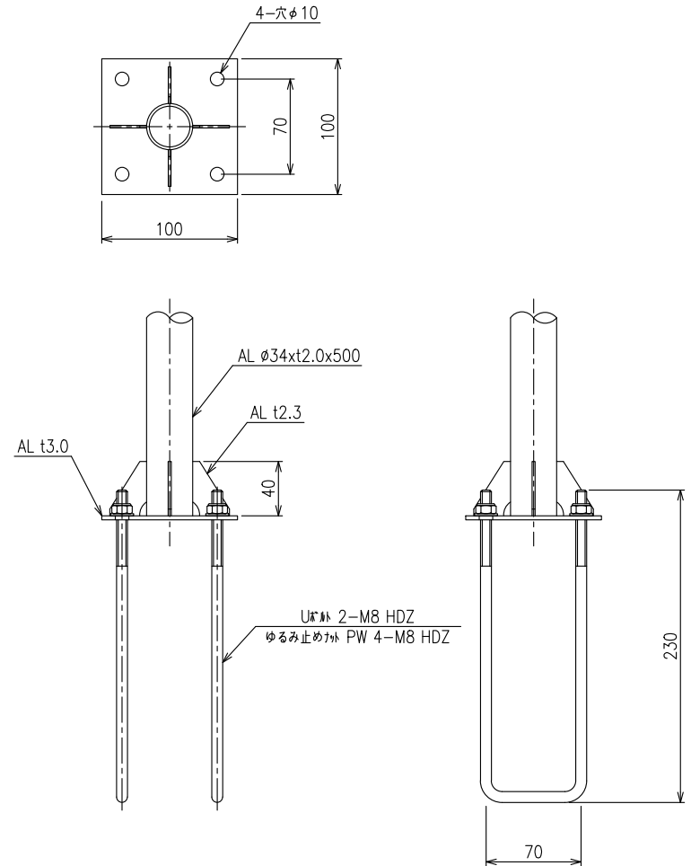
金具詳細図 S=1:5
